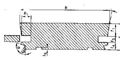
FIG. 2 - Elemento tipo 2
